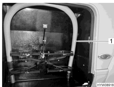
Fig. 207 Tubo di gomma per lo scarico (vano portabombole)
