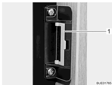
Bild 100 Låsanordning (normalläge)
