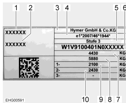
Obr. 186 Typový štítek
