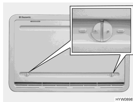
Obr. 148 Zimní kryt (větrací mřížka ledničky)
