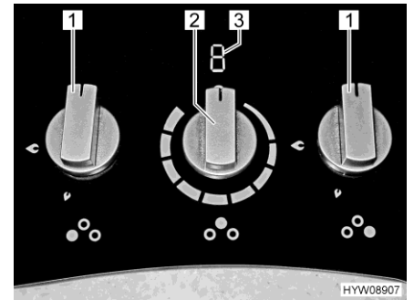
Fig. 199 Elementos de mando (cocina de gas con placa de inducción)
