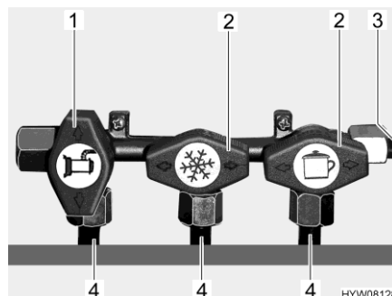
Fig. 132 Posición de las válvulas de paso de gas (ejemplo)
