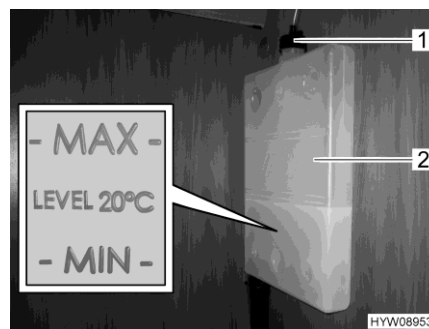
Obr. 229 Značka "MIN/MAX"
