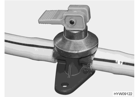
Obr. 178 Vypouštěcí kohout (bojler Alde)
