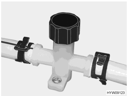
Fig. 215 Robinet de vidange (conduite d'eau)
