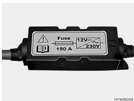
Fig. 152 Fusible (onduleur (150 A))
