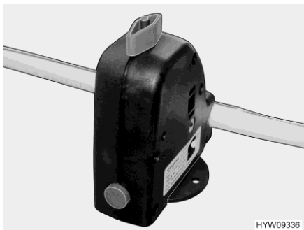
Fig. 216 Valve de sécurité et de vidange (Truma)
