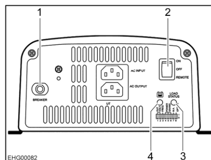
Fig. 139 Onduleur (exemple de représentation)
