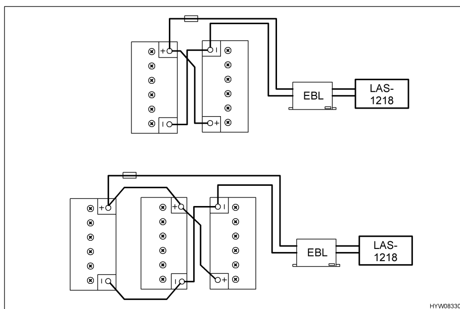
Fig. 132 Brancher la batterie supplémentaire
