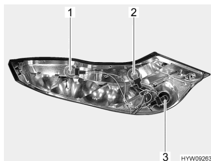
Fig. 232 Unité de feux arrière (démontée)
