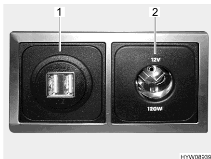
Fig. 129 Prise USB et prise de courant 12 V
