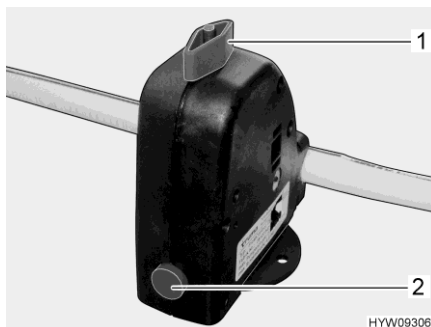
Fig. 163 Valve de sécurité et de vidange (chauffe-eau)
