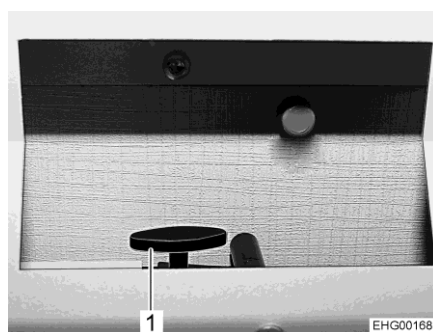
Fig. 165 Papillon (ouvert)
