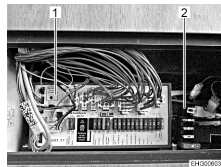
Fig. 146 Bloc électrique EBL 402 et porte-fusible
