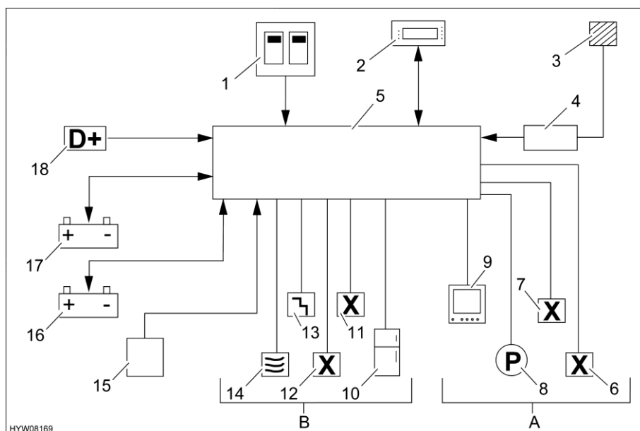
Fig. 157 Schéma du plan des circuits de 12 V
