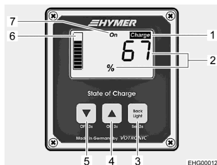
Fig. 133 Panneau d'affichage (indication de l'état de charge total)
