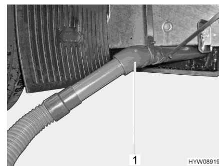
Fig. 207 Tuyau de purge avec tuyau d'évacuation des eaux usées
