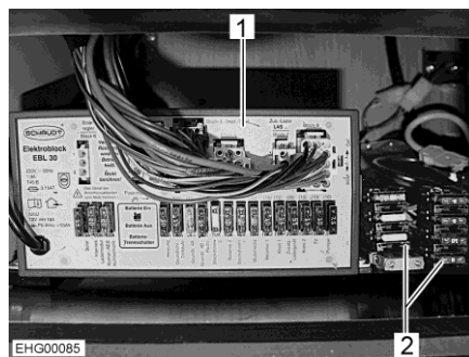
Fig. 145 Bloc électrique EBL 30 et porte-fusible
