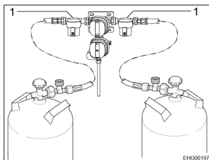
Fig. 127 Filtre à gaz
