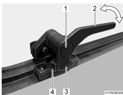
Fig. 57 Levier de verrouillage (position "Fermé")
