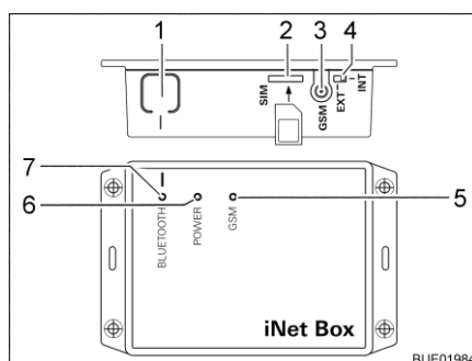
Fig. 186 Truma iNet-Box
