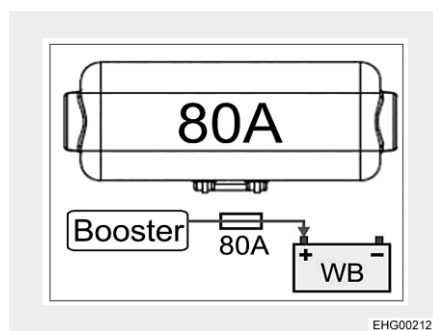
Fig. 150 Fusibles de la batterie de cellule (WB)
