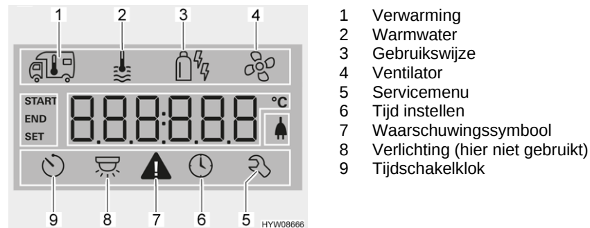
Afb. 160 Display (bedieningspaneel)
