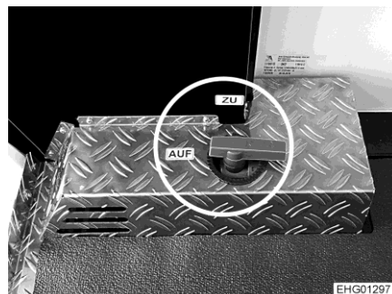
Afb. 205 Bedieningshendel (aftapkraan)
