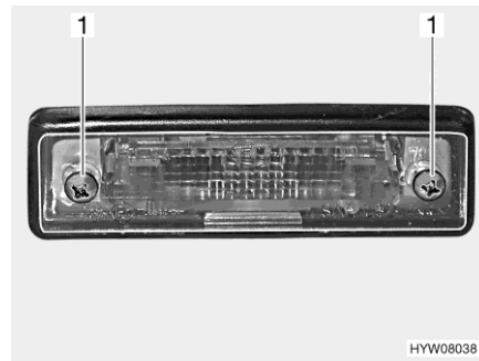
Afb. 235 Verlichting achter (kentekenplaatlampje)
