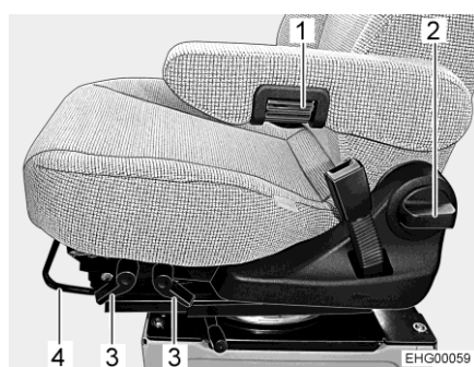
Afb. 22 Stoelverstelling (Aguti GIS-Liner)
