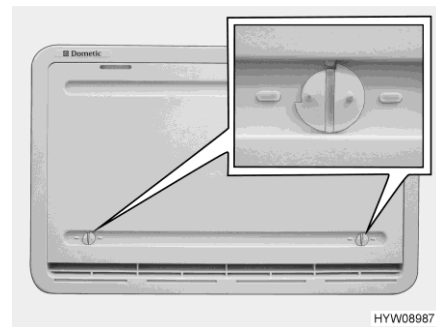
Afb. 194 Winterafdekking (koelkast-ventilatie-rooster)
