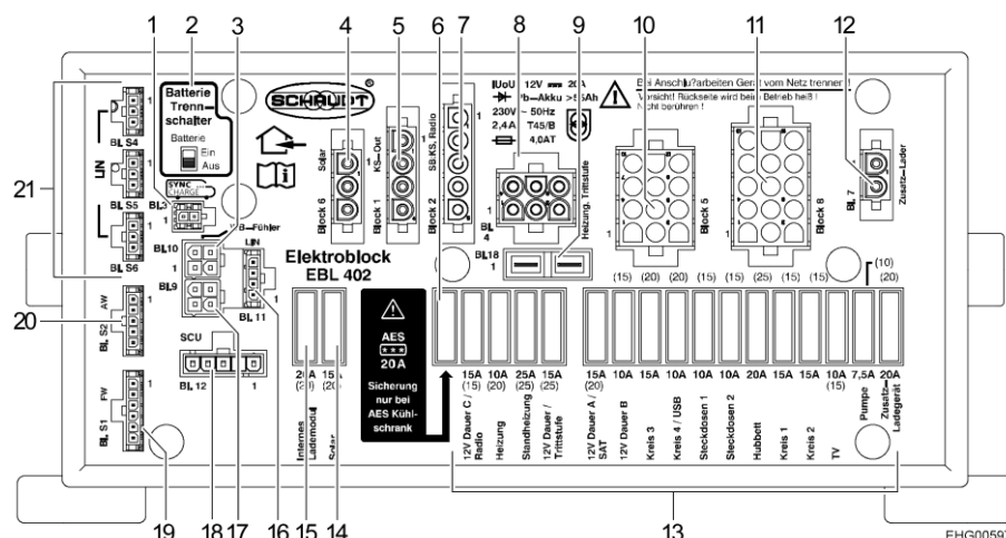
Afb. 139 Elektroblok (EBL 402)
