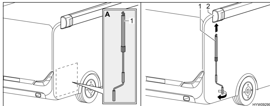
Afb. 49 Slinger aanbrengen
