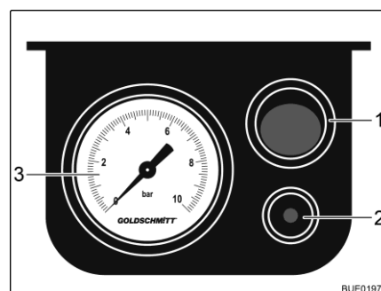
Afb. 15 Elektrisch bedieningsgedeelte
