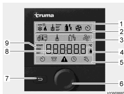
Afb. 165 Bedieningspaneel met displays
