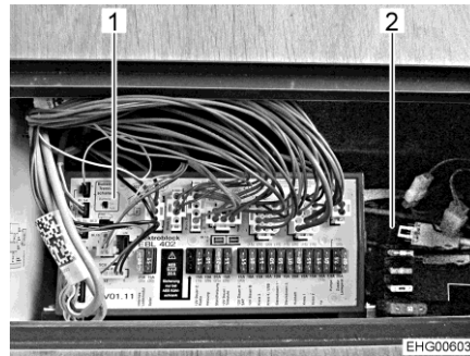
Afb. 149 Elektroblok EBL 402 en zekeringhouders
