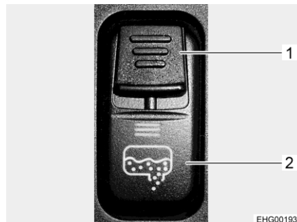
Afb. 204 Wipschakelaar (voor af laten lopen van afvalwater)
