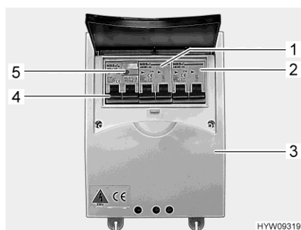
Afb. 146 Beveiligingsautomaat en FI-schakelaar (230-V-zekeringenkast)
