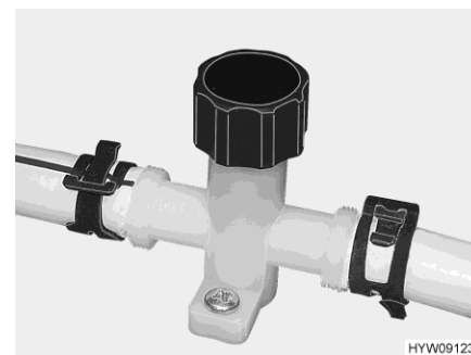
Afb. 217 Aftapkraan (waterleiding)
