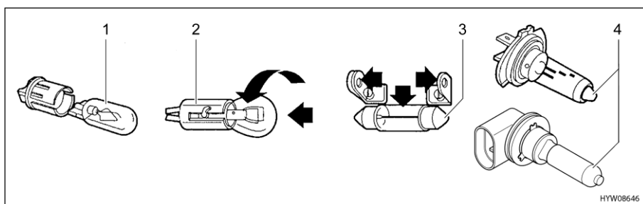
Afb. 226 Gloeilamptypen
