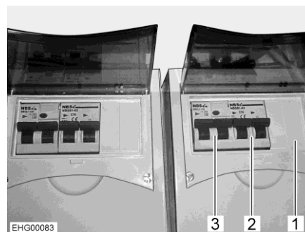
Afb. 144 Extra zekeringenkasten
