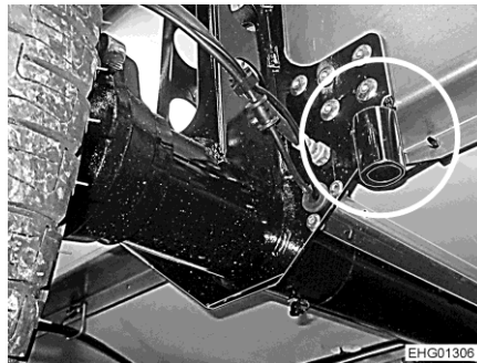
Afb. 242 Houder achteras
