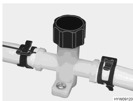
Afb. 200 Aftapkraan (waterleiding)
