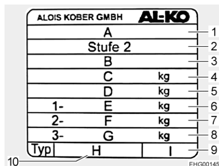
Afb. 238 Typeplaatje chassis
