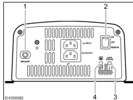
Afb. 143 Wisselrichter (voorbeeldweergave)
