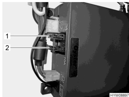
Afb. 153 Besturingsapparaat (TV-satellietinstallatie)
