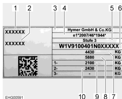
Afb. 237 Typeplaatje
