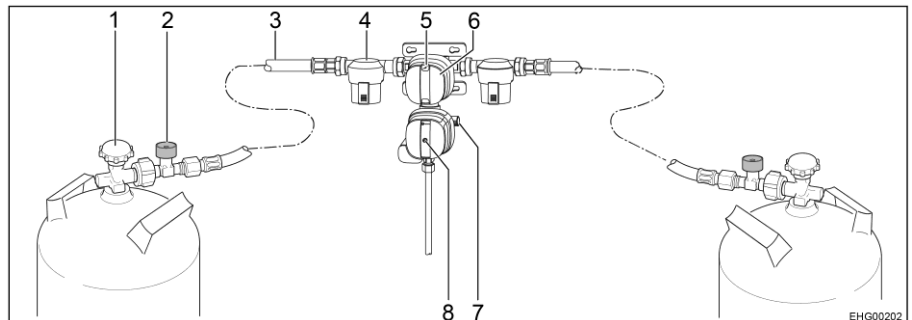
Afb. 132 Veiligheidsgasdrukregelaar DuoControl CS
