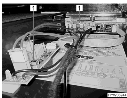
Afb. 151 Zekeringen (warmwaterverwarming)
