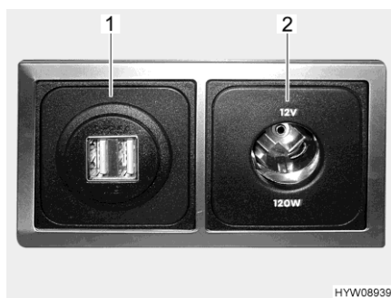
Fig. 87 Combinaison prise de courant USB et 12 V (exemple)
