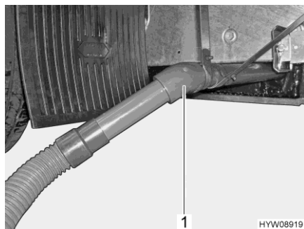
Fig. 155 Tuyau de purge avec tuyau d'évacuation des eaux usées
