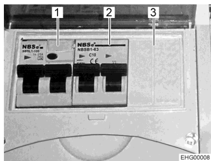
Fig. 94 Coffret de fusibles supplémentaire
