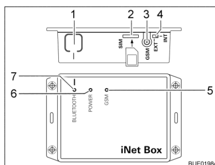
Fig. 116 Truma iNet-Box
