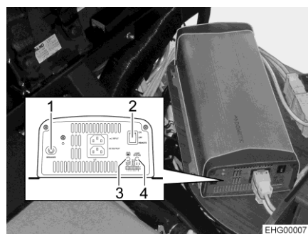
Fig. 93 Onduleur (exemple de représentation)
