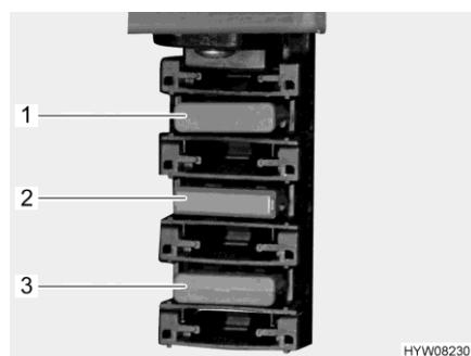
Fig. 100 Fusibles (porte-fusibles)
