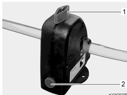
Fig. 148 Valve de sécurité et de vidange (Truma)
