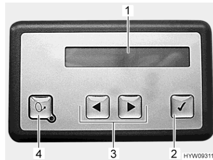
Fig. 62 Unité de commande (antenne parabolique)
