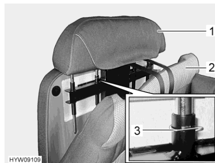
Fig. 18 Régler l'appuie-tête
