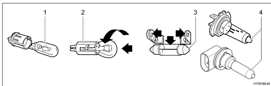
Fig. 175 Types d'ampoules
