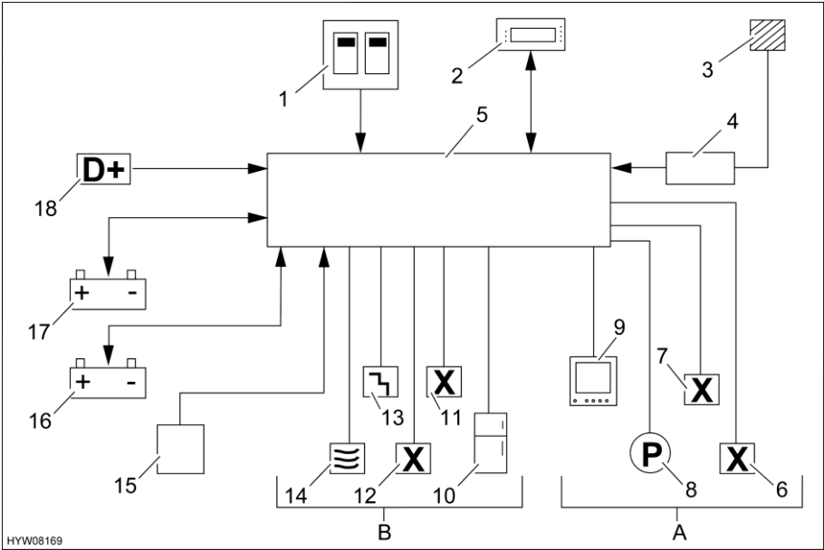
Fig. 108 Schéma du plan des circuits de 12 V
