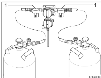
Fig. 85 Filtre à gaz
