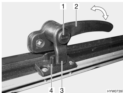
Fig. 35 Levier de verrouillage (position "Fermé")
