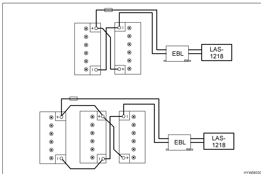
Fig. 89 Brancher la batterie supplémentaire
