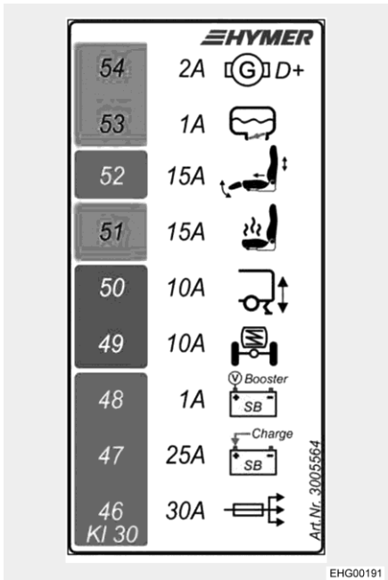
Fig. 103 Fusibles console du siège conducteur
