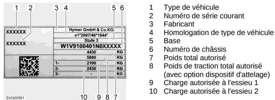
Fig. 180 Plaque signalétique
