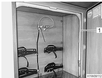
Fig. 153 Tuyau d'évacuation des eaux usées (compartiment à gaz)
