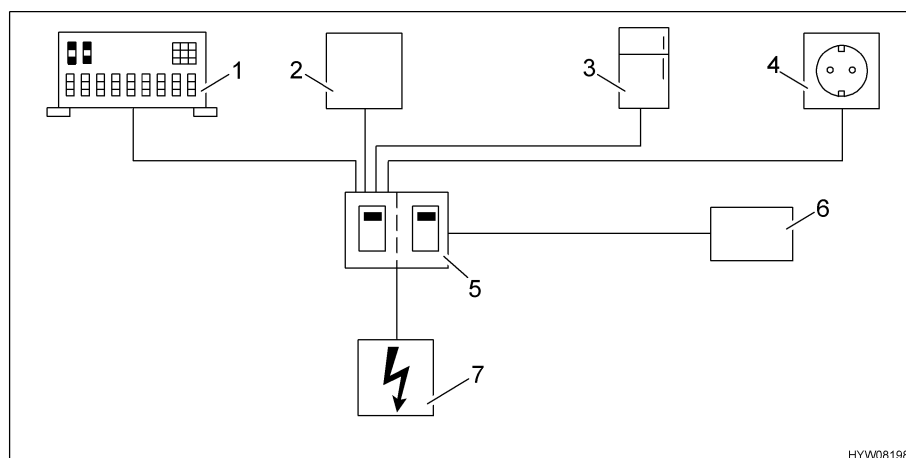
Fig. 107 Schéma du plan des circuits de 230 V
