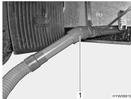
Afb. 155 Afvoerbuis met afvalwaterslang
