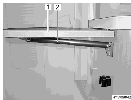
Afb. 57 Vouwtafeltje
