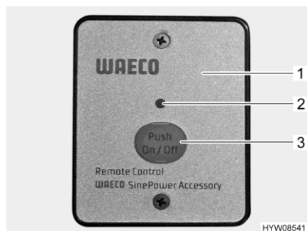
Afb. 95 Externe schakelaar (wissel- richter)
