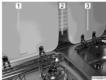
Afb. 9 Vlambeschermingsplaat en afdekkingen
