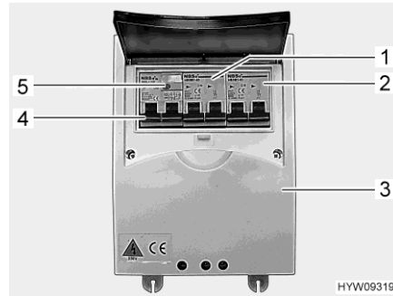
Afb. 97 Beveiligingsautomaat en FI-schakelaar (230-V-zekeringenkast)
