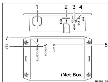
Afb. 116 Truma iNet-Box
