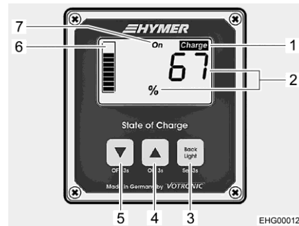
Afb. 90 Display (aanduiding totale laadtoestand)
