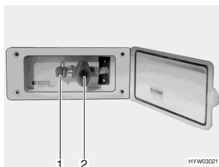
Afb. 79 Externe gasaansluiting (gasafsluitkraan gesloten)
