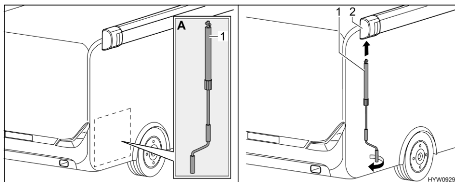
Afb. 25 Slinger aanbrengen
