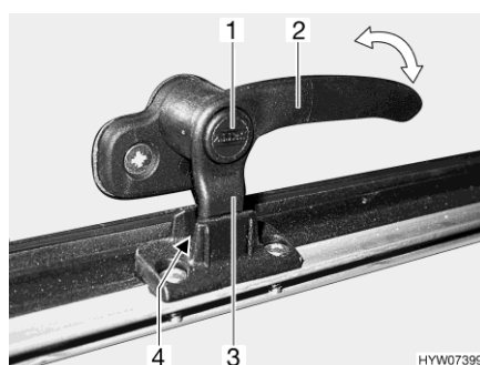
Afb. 37 Vergrendelingshendel (stand "continue ventilatie")
