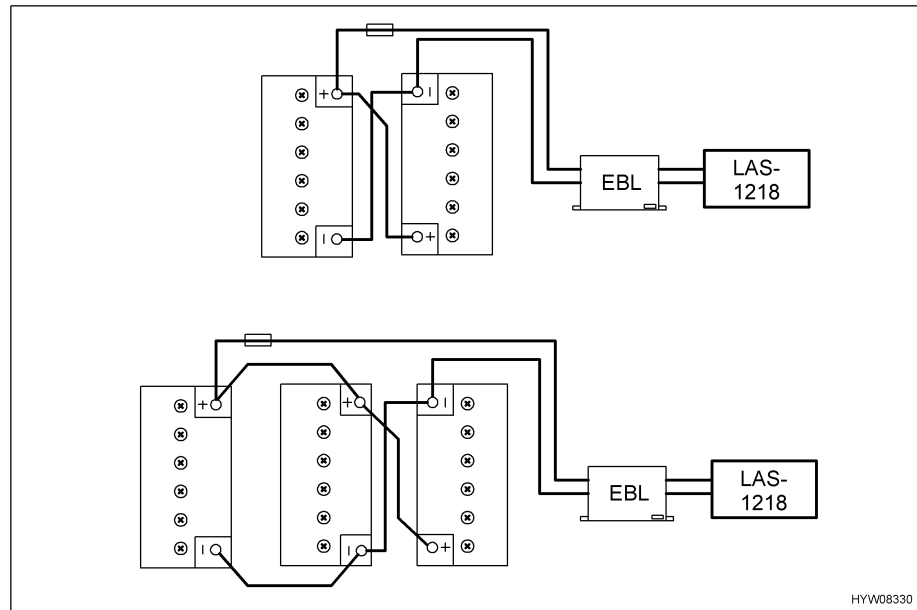
Afb. 89 Extra accu aansluiten
