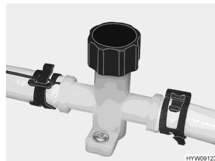
Afb. 167 Aftapkraan (waterleiding)
