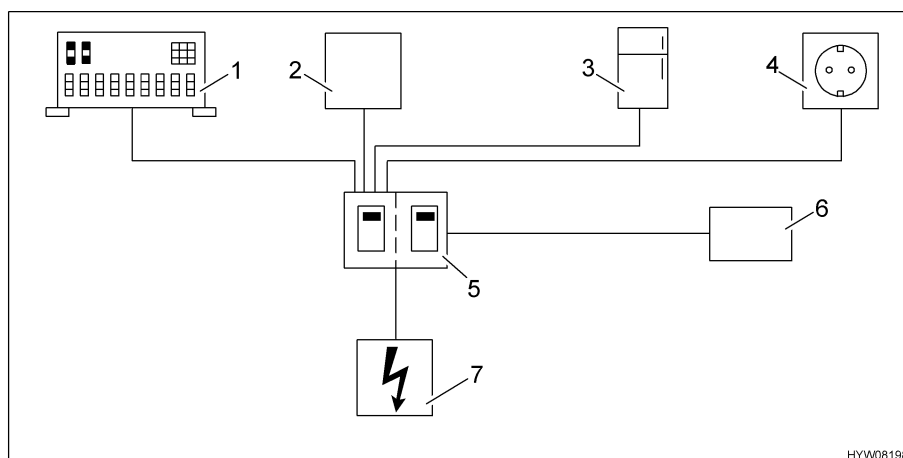
Afb. 107 Schema 230-V-bedrading
