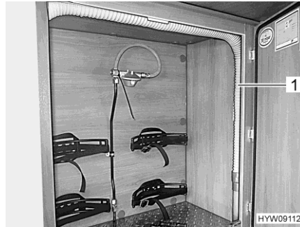
Afb. 153 Afvalwaterslang (gaskast)
