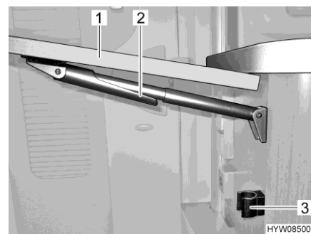
Afb. 58 Vouwtafeltje wegklappen
