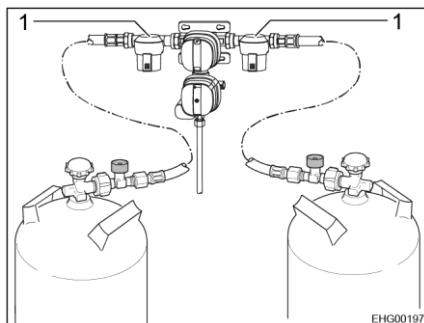
Afb. 85 Gasfilter
