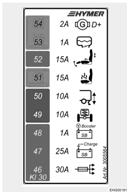
Afb. 103 Zekeringen console van de bestuurdersstoel
