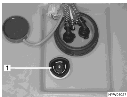
Afb. 152 Draaigreep (watertank)
