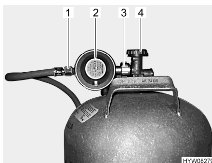
Afb. 86 Aansluiting gasfles
