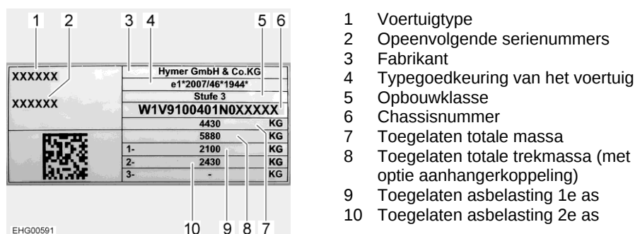
Afb. 180 Typeplaatje
