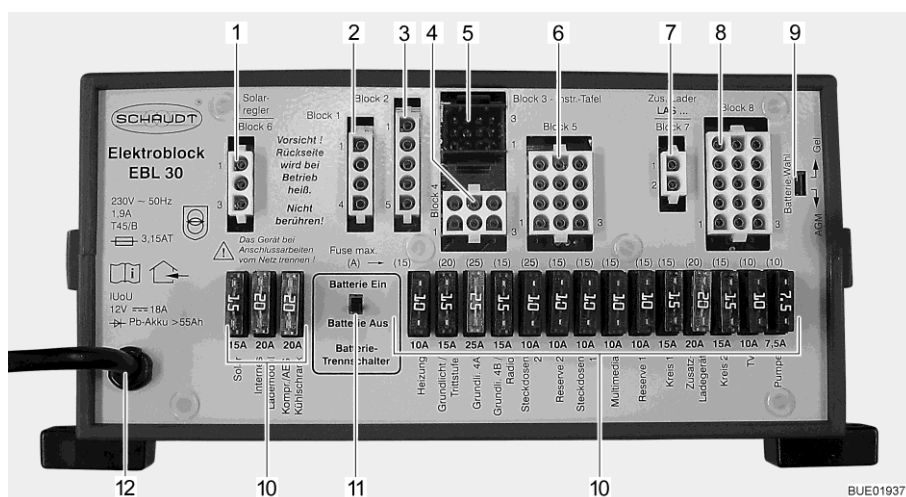
Afb. 92 Elektroblok (EBL 30)
