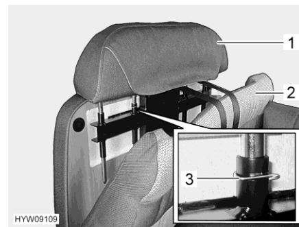
Afb. 18 Hoofdsteun instellen
