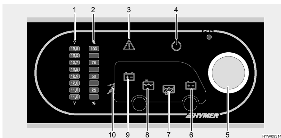
Afb. 96 Paneel (LT 94)
