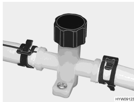
Afb. 120 Aftapkraan (waterleiding)
