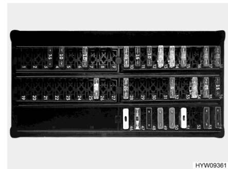
Afb. 102 Zekeringen (linkerstoelconsole)
